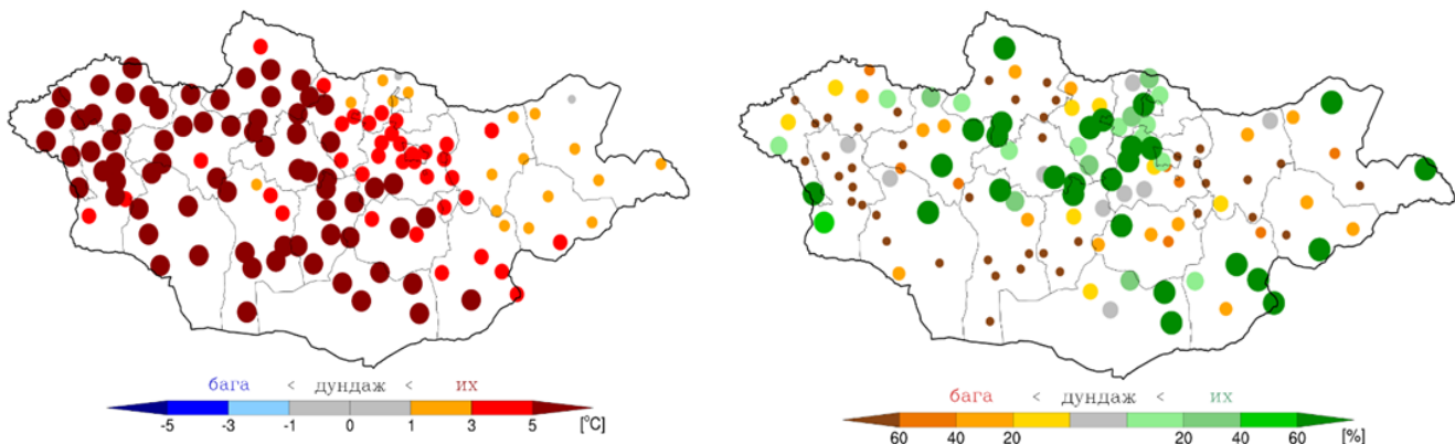
Зураг 2. 2021 оны 2 дугаар сарын агаарын дундаж температур, нийлбэр хур тунадасны ОЖД-аас хазайх хазайлтын газарзүйн тархалт
