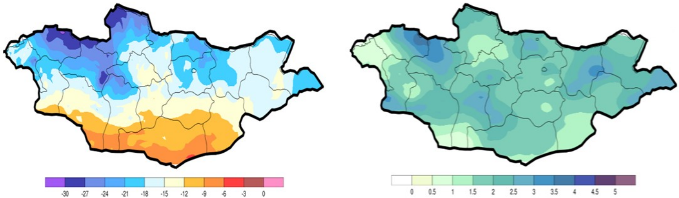
Зураг 1. 1981-2010 оны 2 дугаар сарын агаарын дундаж температур, нийлбэр хур тунадасны газарзүйн тархалт
