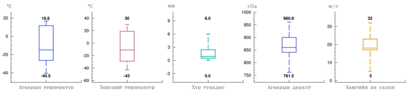
Зураг 4. Тус сард ажиглагдсан экстремаль утгууд
